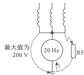
图 1 发电机中性点注入电压的原理
