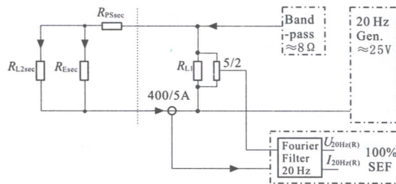
图 3 100% 定子接地保护等效回路
